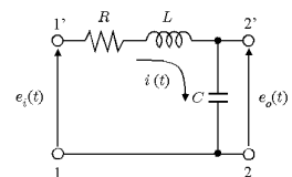
図 2.4 RLC回路
