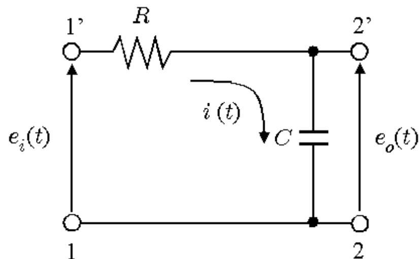
図 2.8 RC回路
