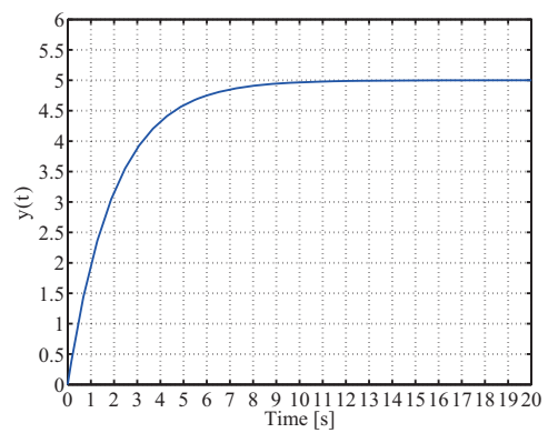
図 1: ステップ応答
