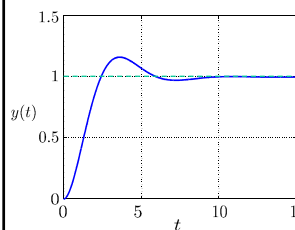
(a) 安定なシステムの応答
