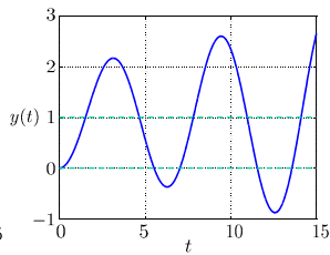
(b) 不安定なシステムの応答
