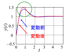
図 9.2 (b) 目標値応答 (r=1) 6
