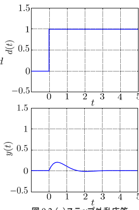
図 9.2 (a) ステップ外乱応答
