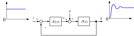
図 9.1 フィードバック制御系
