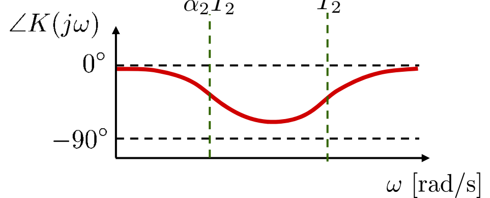
図8.10 位相遅れ補償のボード線図
