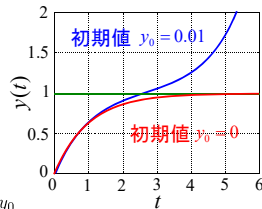
図 6.2 ステップ応答例
