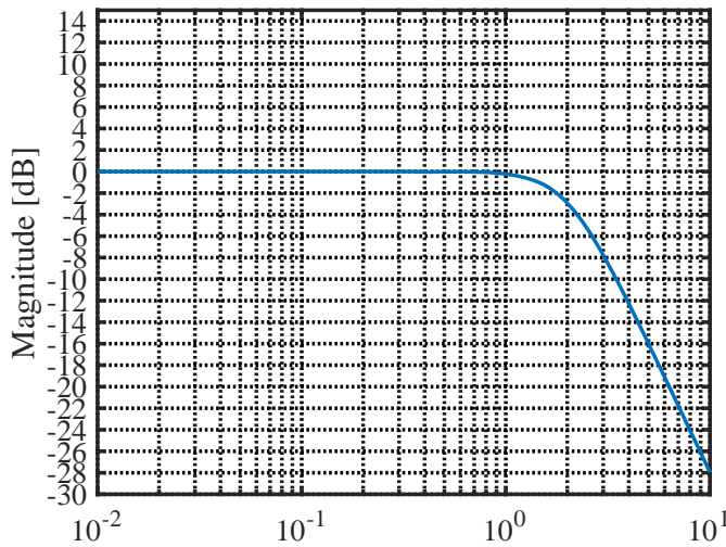
図 1-1: ボード線図
